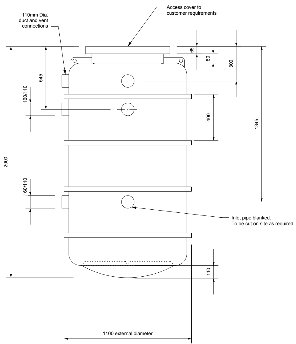
END ELEVATION
