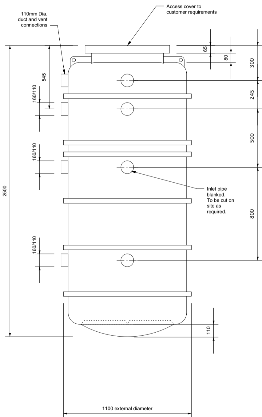
END ELEVATION
