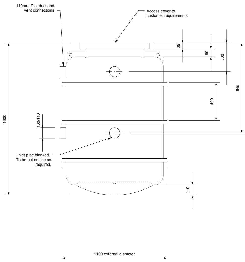
END ELEVATION
