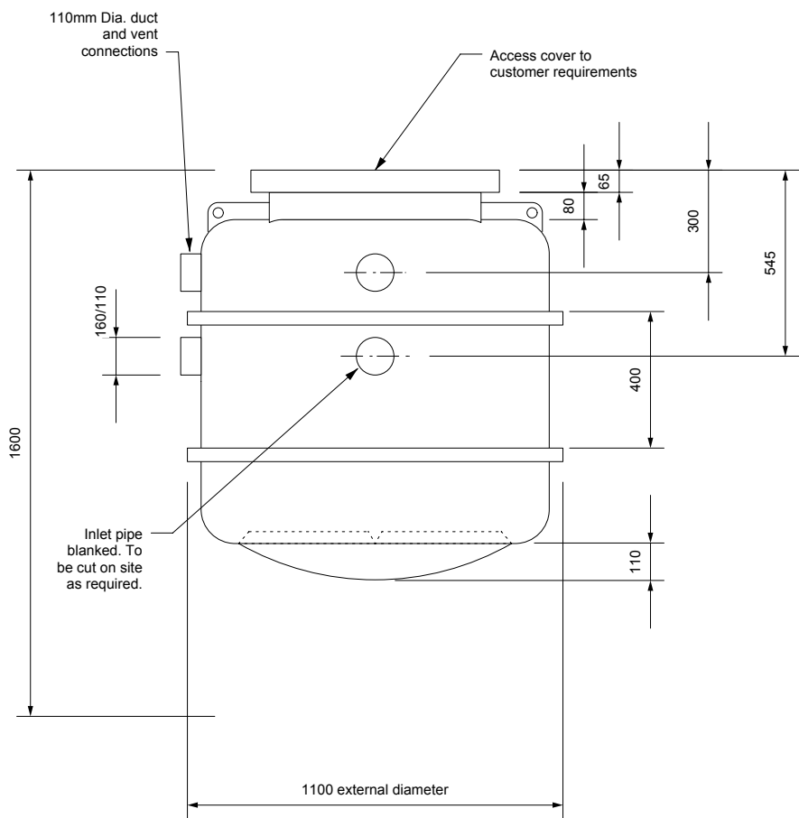
END ELEVATION
