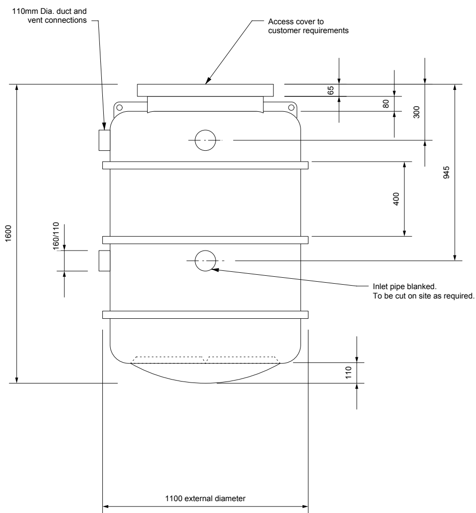
END ELEVATION
