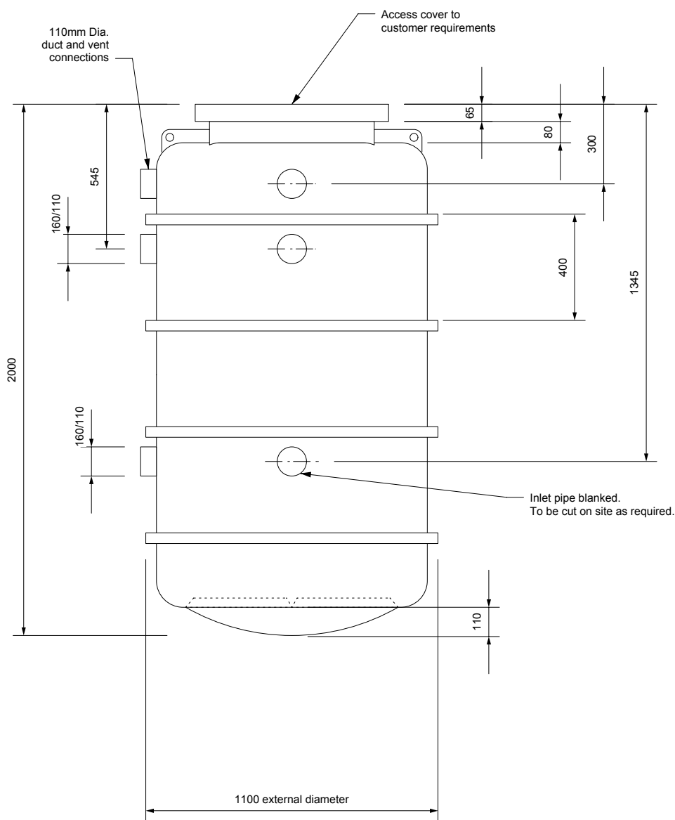
END ELEVATION
