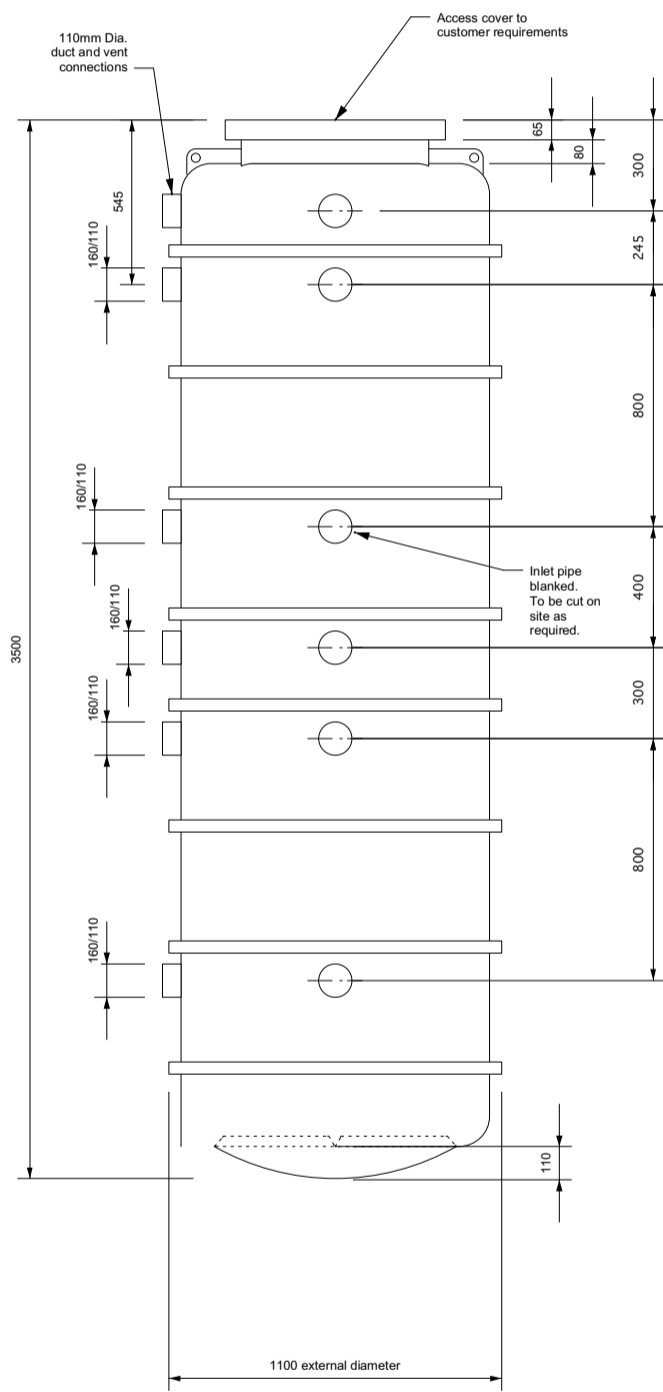
END ELEVATION
