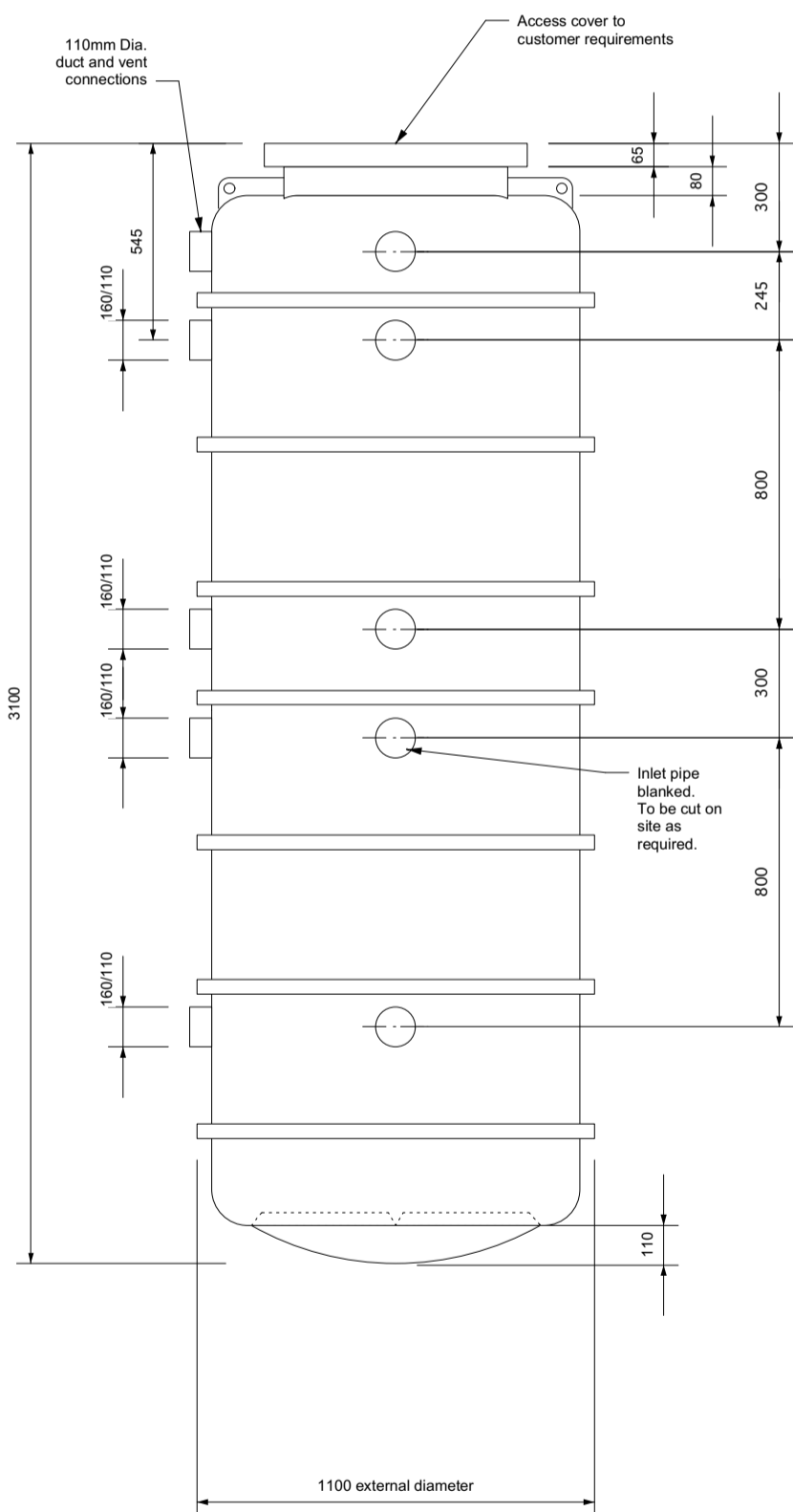
END ELEVATION
