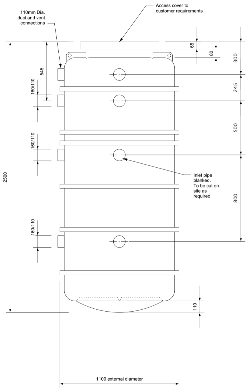
END ELEVATION
