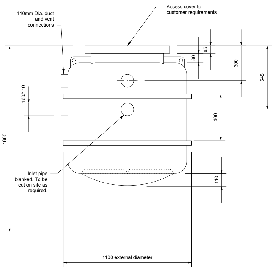
END ELEVATION
